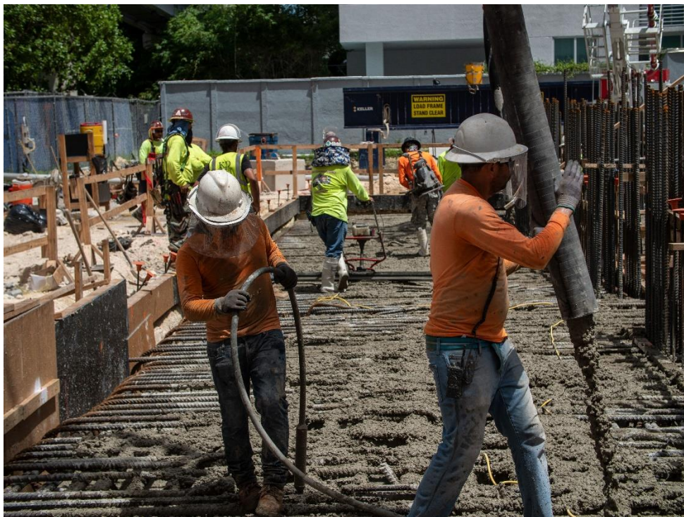
YOTELPAD MIAMI, CEMENT POUR IN ACTION, IMAGE VIA LUIS CARMONA
